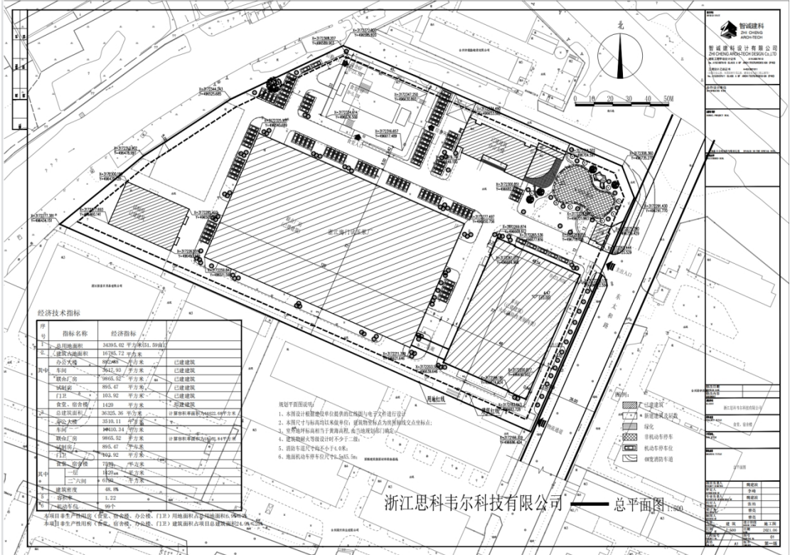
图 3.4 平面布局图
